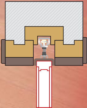
DETALLE SECCIÓN B
