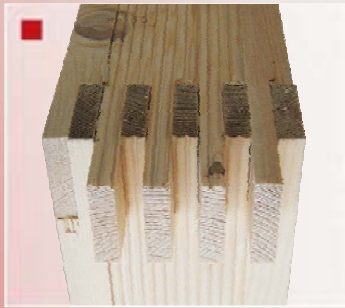
Sistema de mechonado
